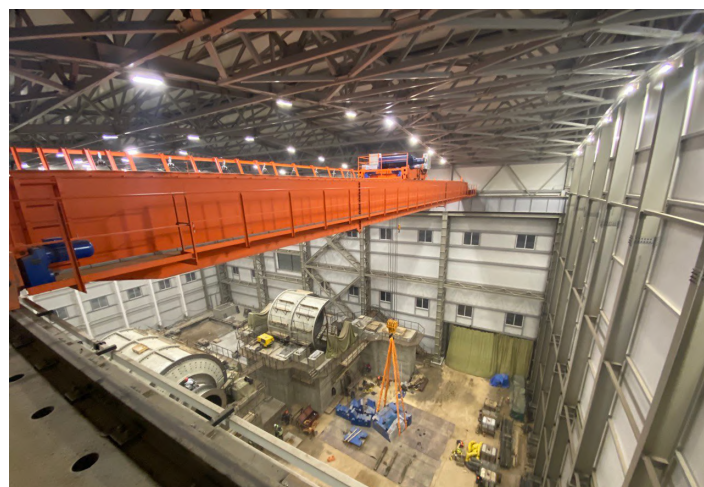
Кран мостовой опорный двухбалочный с электроприводом грузоподъемностью 65,0/5,0 тонн и длиной пролета 36,0 метров для предприятия в Республике Казахстан.
