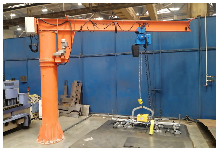
Кран консольный на колонне с электроприводом грузоподъемностью 1,0 тонна для предприятия в г. Набережные Челны.
